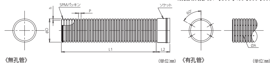
《無孔管》
